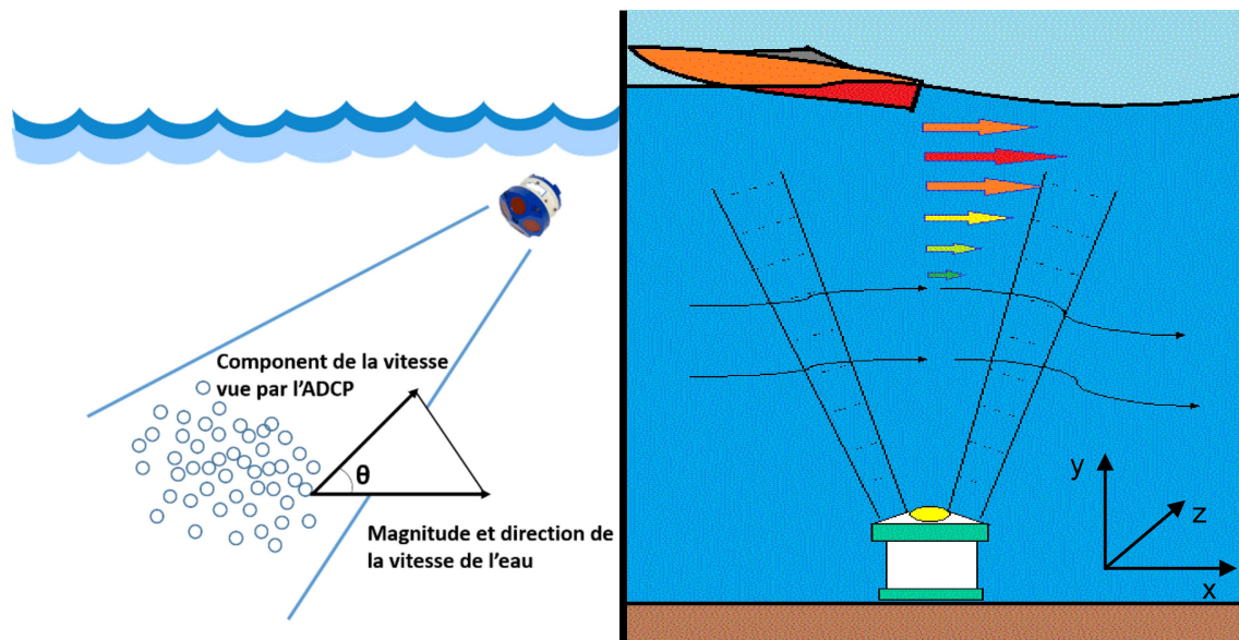
Figure 5: Mesures de courant en 3 dimensions (RD Instrument, 1989)
